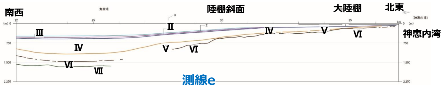
<地質断面図>
