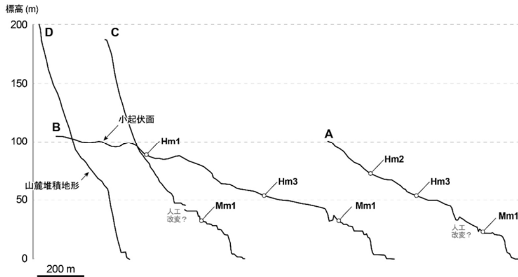
図 4.1-4 海岸部の地形断面
