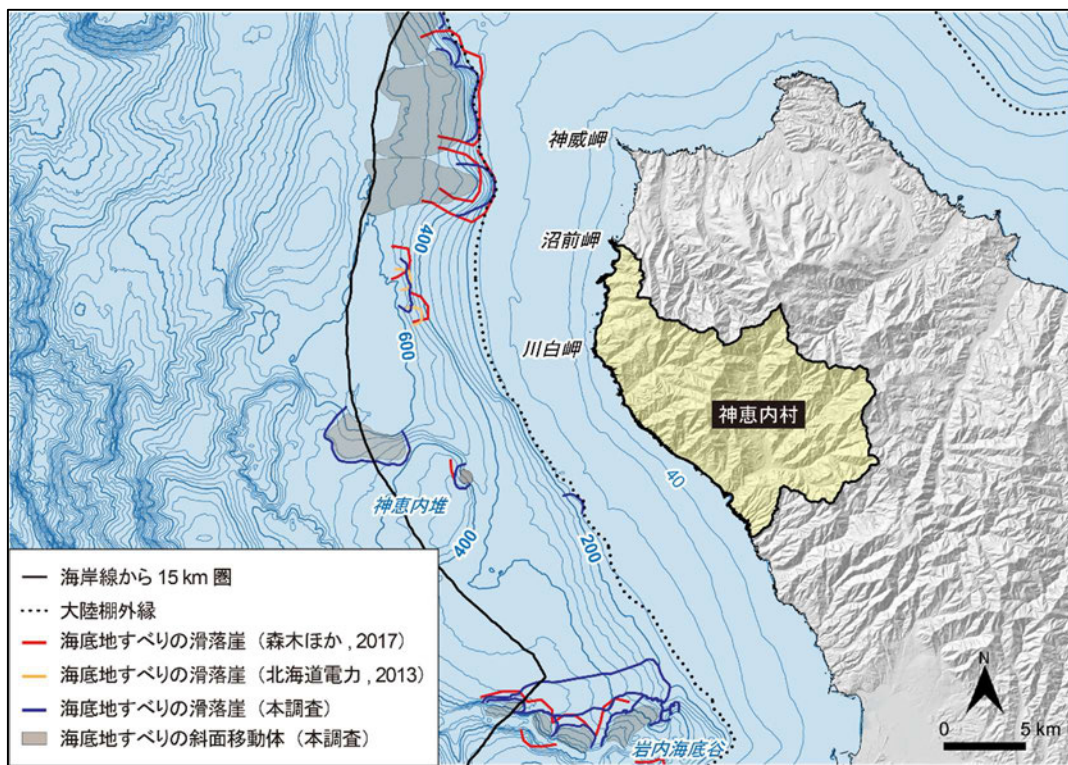
図 4.2-5 文献調査対象地区 (海域) とその周辺地域における海底マスマーブメント地形の分布 図 3.2-4 に本調査による判読結果を重ね合わせた。地理院タイルの陰影起伏図を使用。海域の等深線図は、日本水路協会発行 M7000 シリーズを用いて作成 ((一財) 日本水路協会承認第 2021006 号)。海岸線は「国土数値情報 (海岸線データ)」(国土交通省) に、神恵内村の行政界は「国土数値情報 (行政区域データ)」(国土交通省) に基づく。
