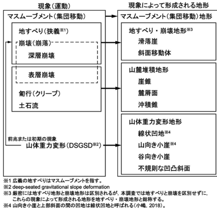
図 4.2-3 マスムーブメントにより形成される地形の概念
