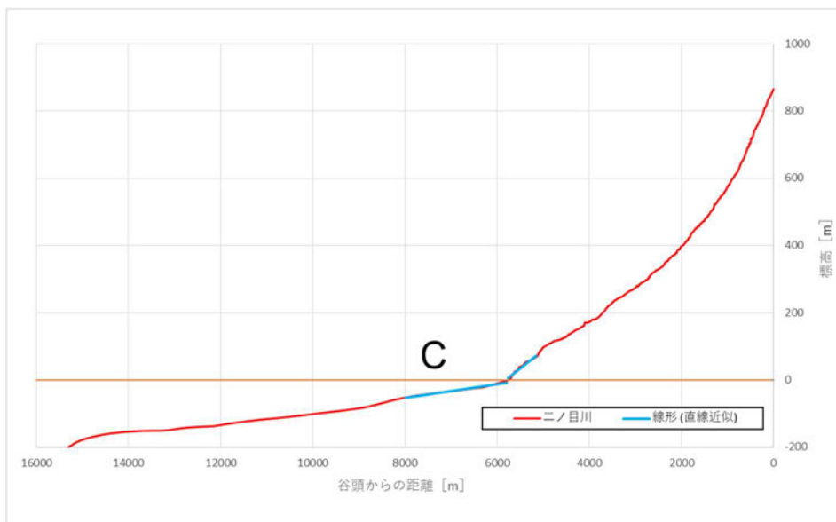
図 D-2 二ノ目川から浅海底にかけての縦断面図
