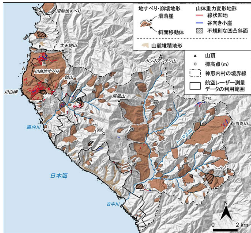
図 4.2-4 文献調査対象地区（陸域）におけるマスマーブメント地形の分布
