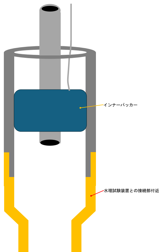
図 2.13.7-2 インナーパッカーの概念図
